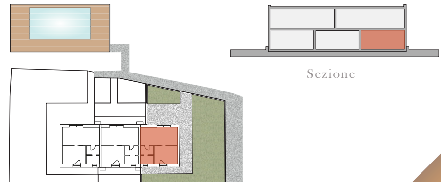
Pianta Edificio
