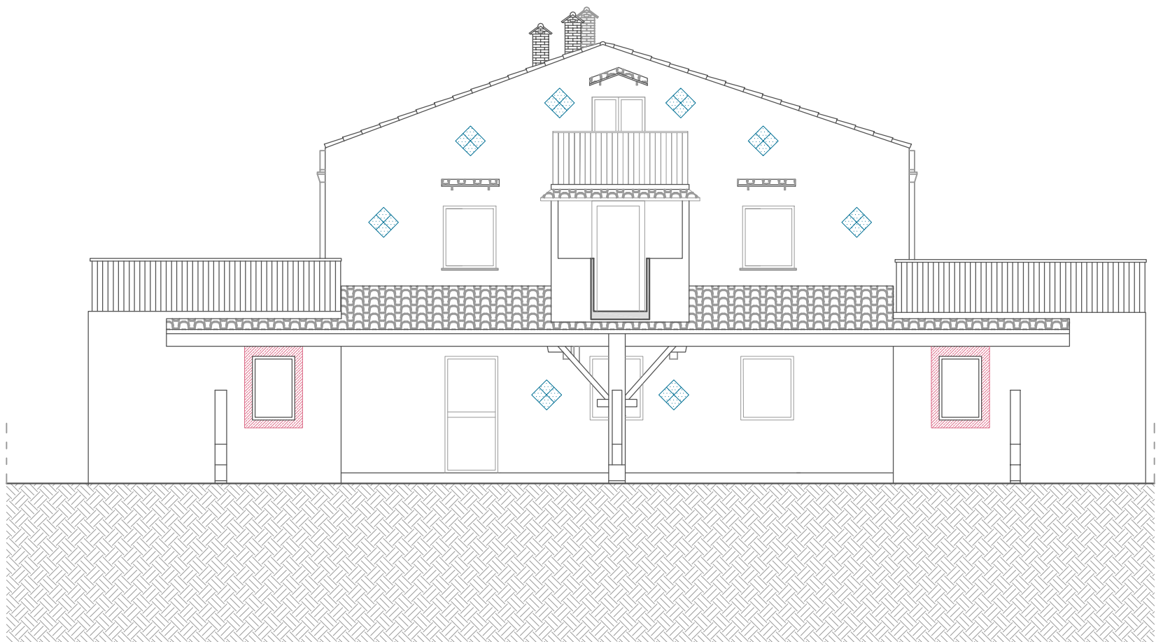
Prospetto Sud
